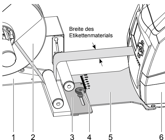
Bild 4 Ausrichten des Aufwicklers zum Drucker
