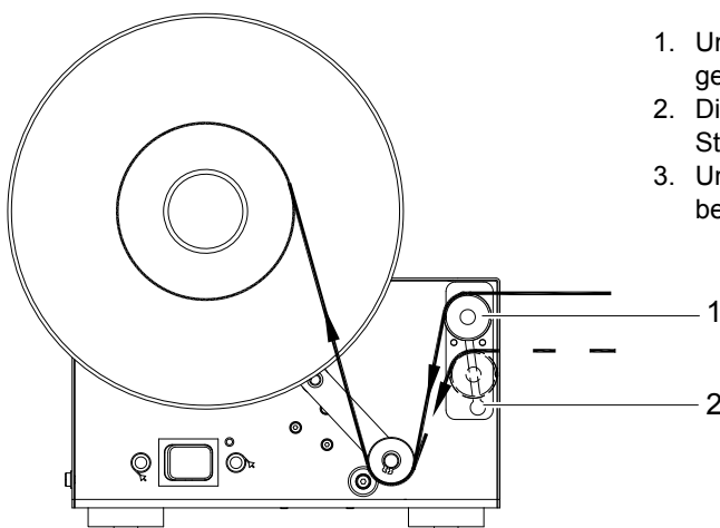
Bild 6 Einstellung der Umlenkachse
