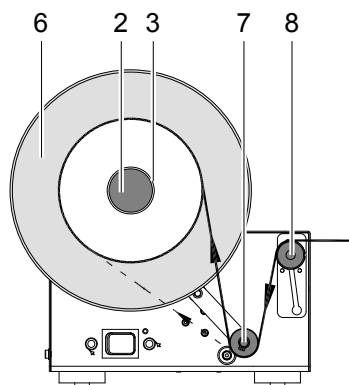
Bild 8 Aufwickeln auf 40-mm-Pappkern (Darstellung unten ohne Teller)
