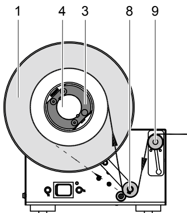
Bild 9 Aufwickeln auf 76-mm-Pappkern (Darstellung unten ohne Teller)
