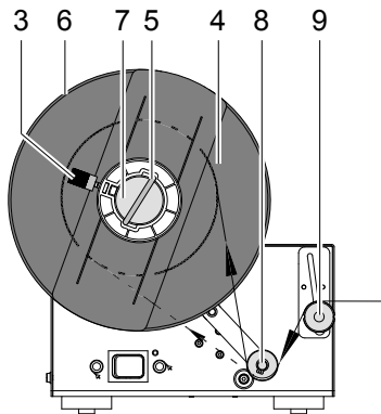
Bild 7 Aufwickeln direkt auf die Wickelachse
